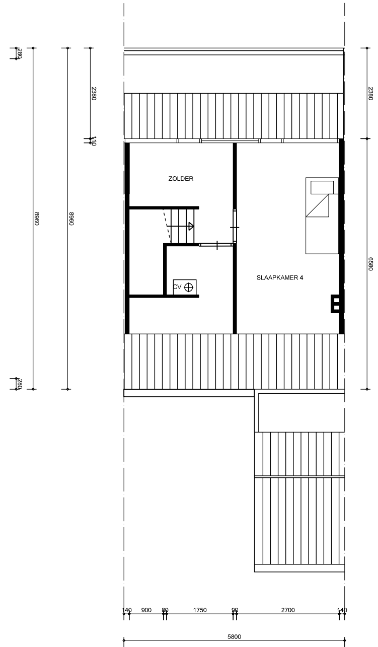
2e VERDIEPING
