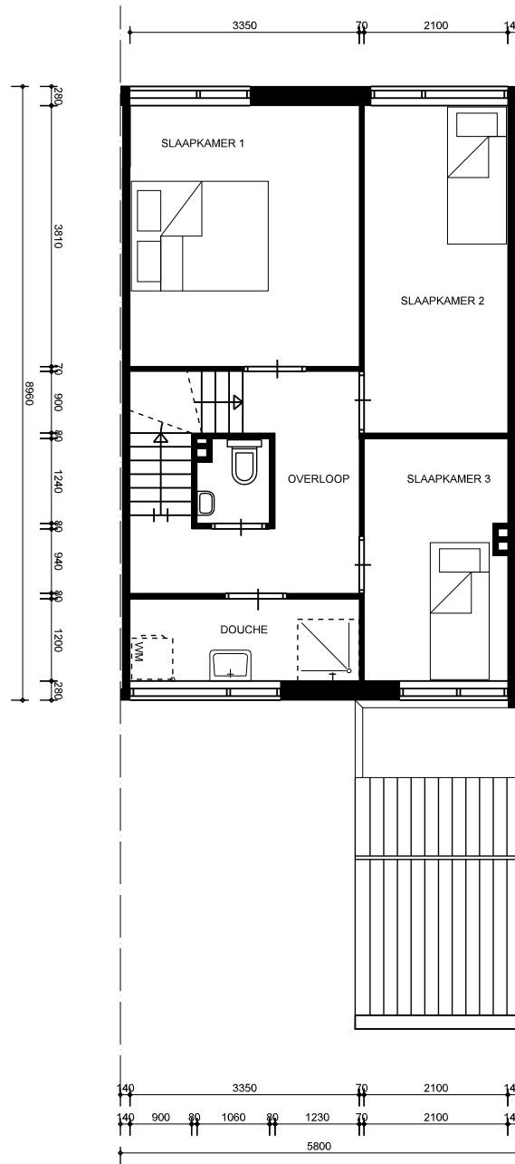
1e VERDIEPING
