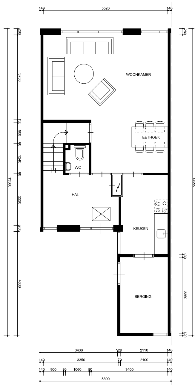
BEGANE GROND
