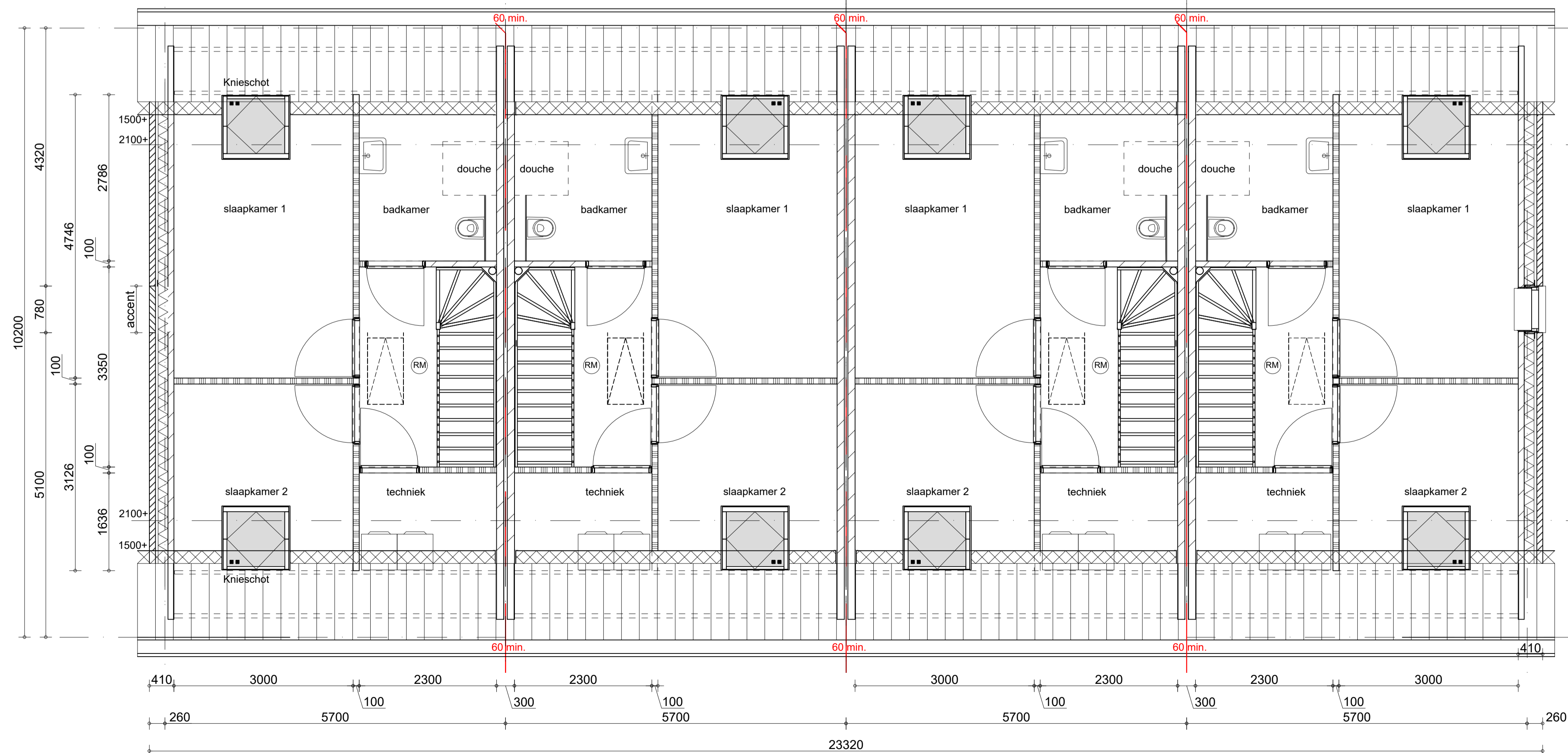
Verdieping 1:50
