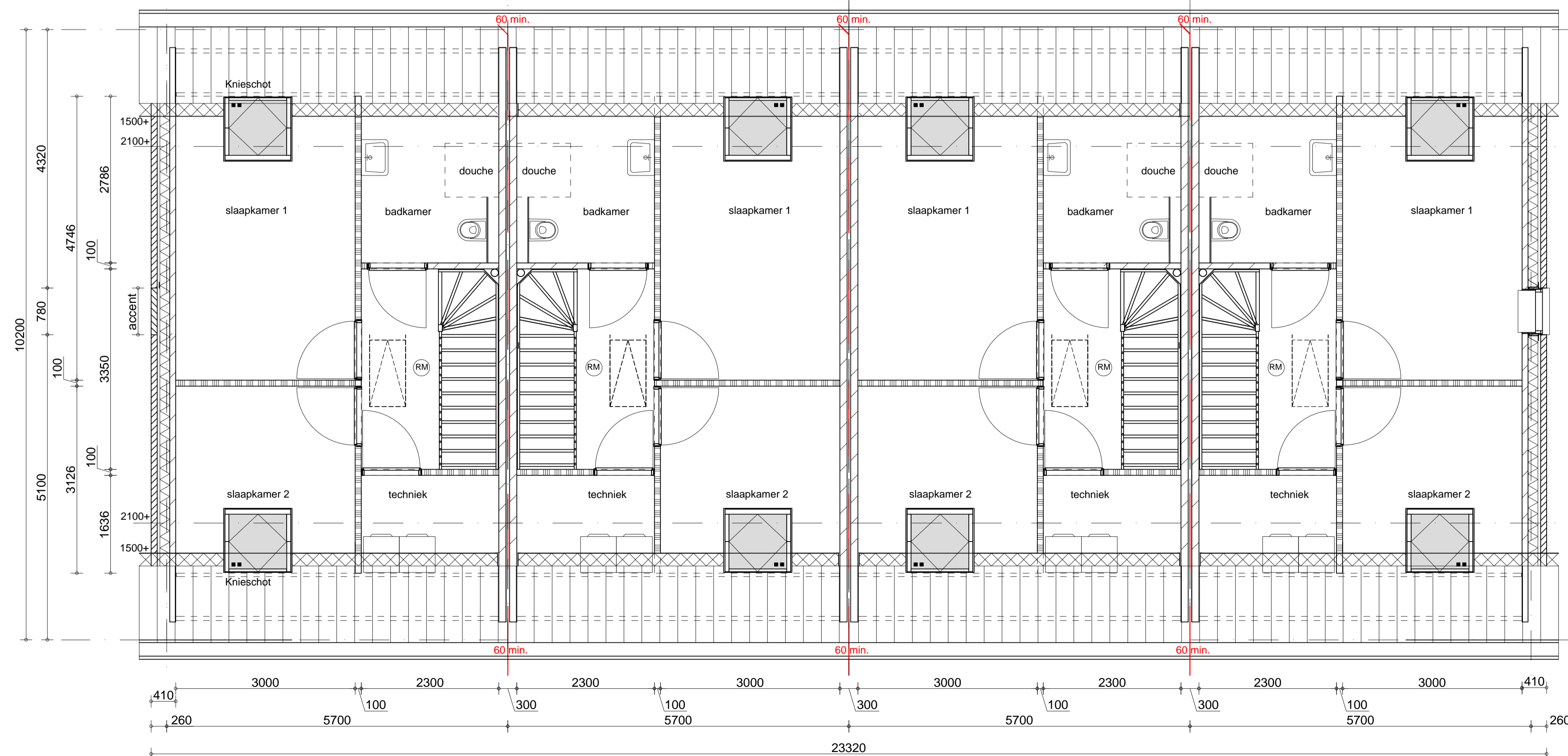
Verdieping 1:50
