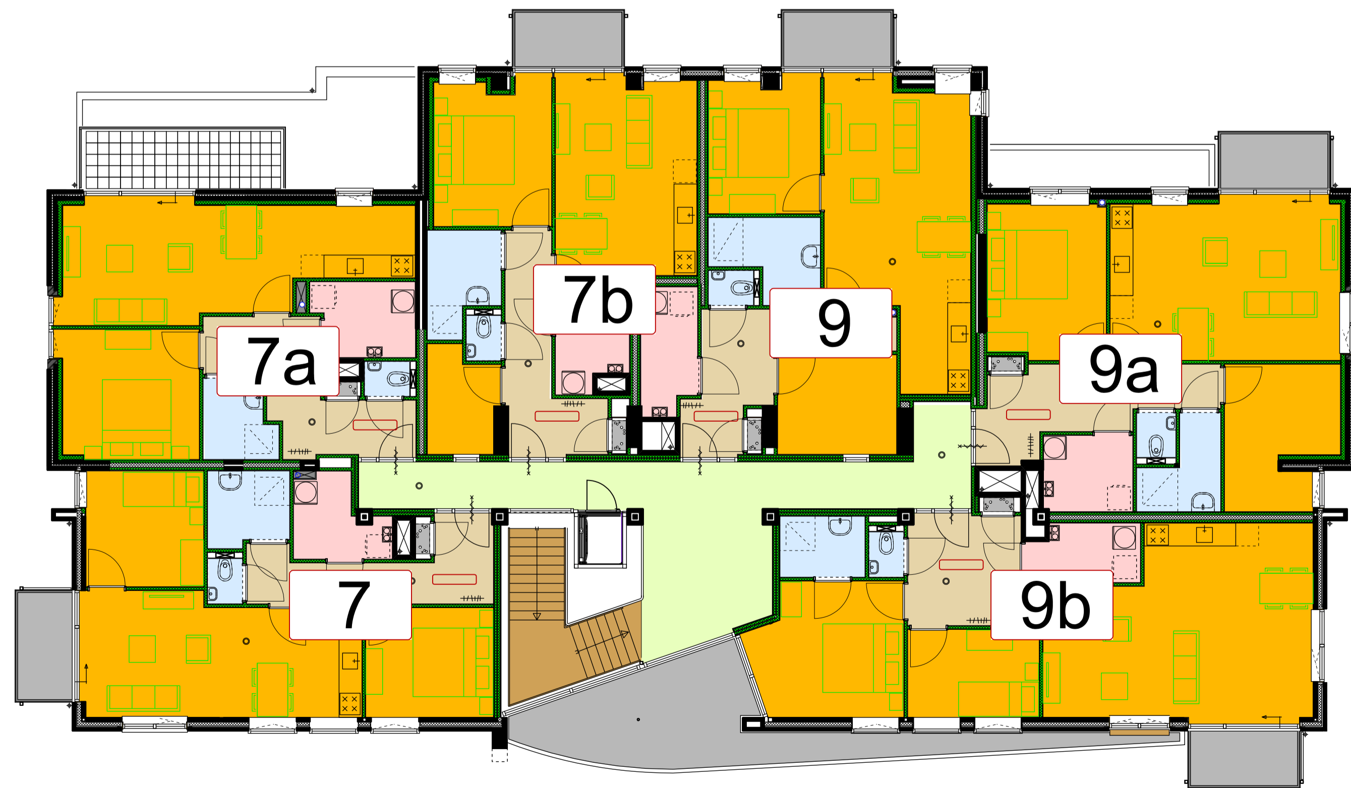
Eerste verdieping
